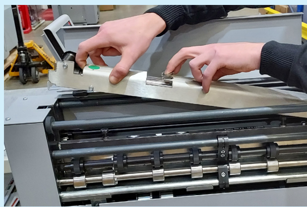
Зняття захисної кришки «EasyBlade».
