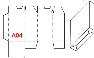
Коробки з нижнім замком блокування
