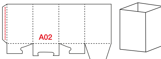
Коробки з замикаючим дном
