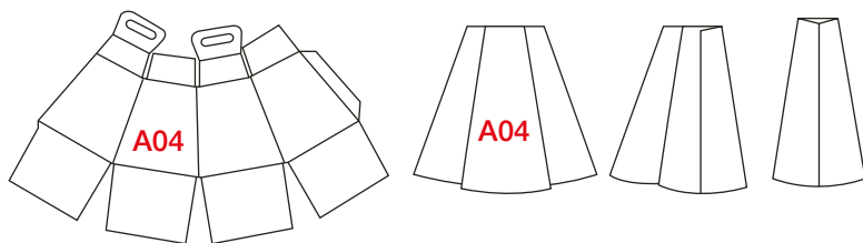
Конічні лінійні коробки
